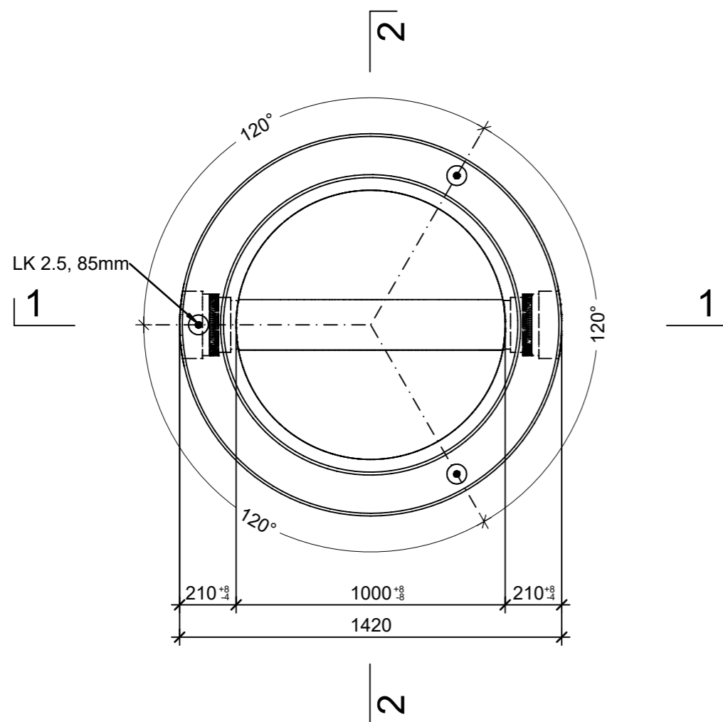
Grundriss, 1:20
