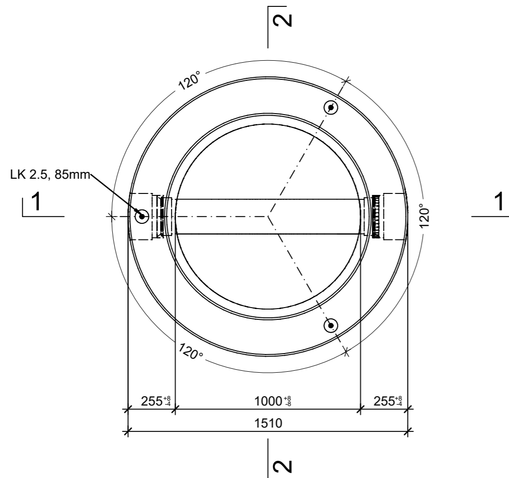
Grundriss, 1:20
