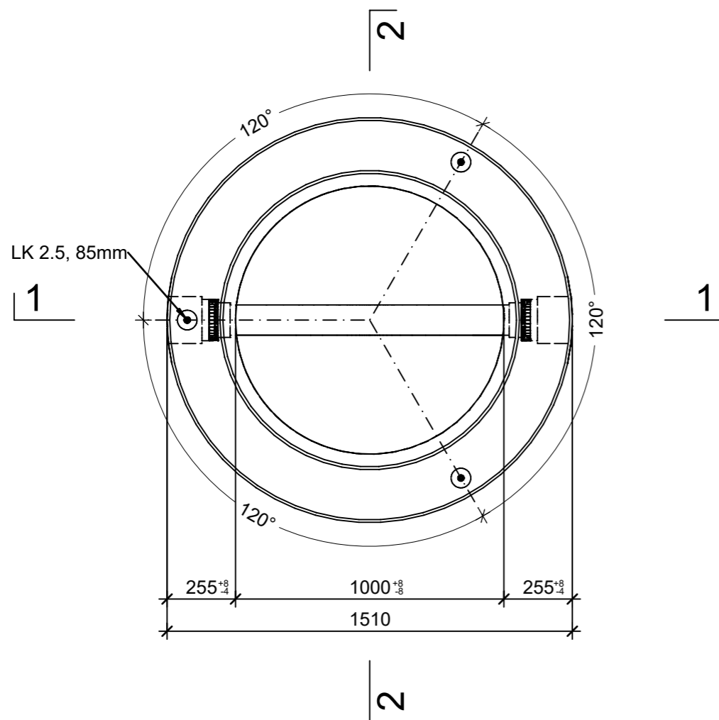
Grundriss, 1:20
