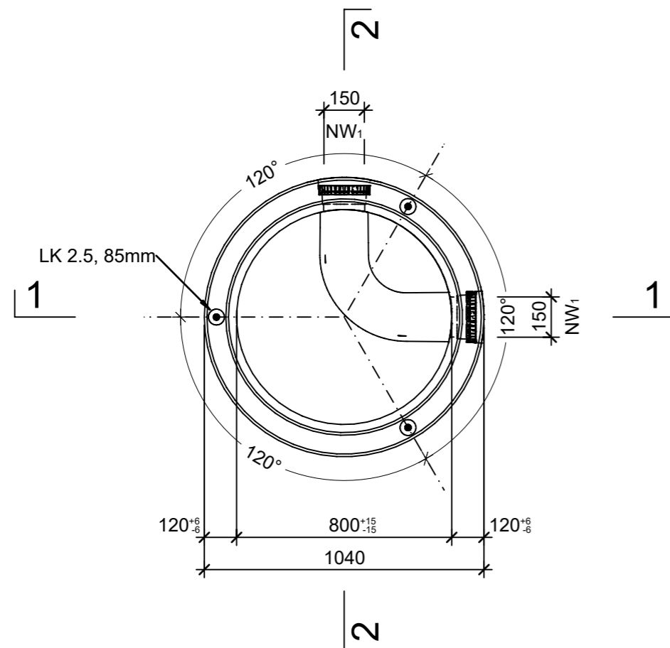
Grundriss, 1:20
