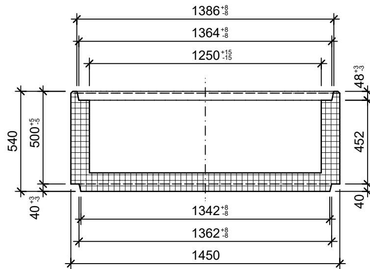
Schnitt 1-1, 1:20
