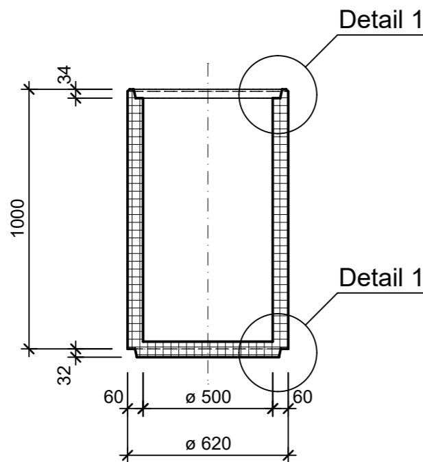
Schnitt A - A, 1:20
