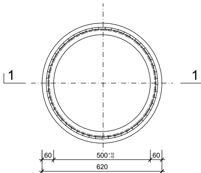
Grundriss, 1:10
