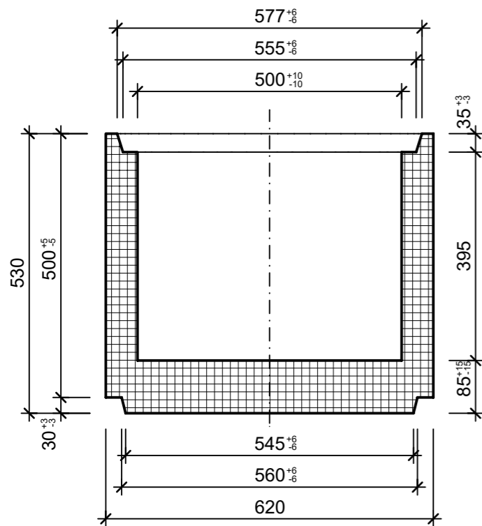
Schnitt 1-1, 1:10
