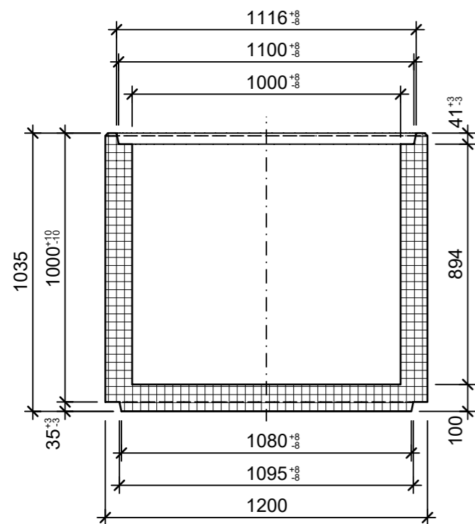
Schnitt 1-1, 1:20
