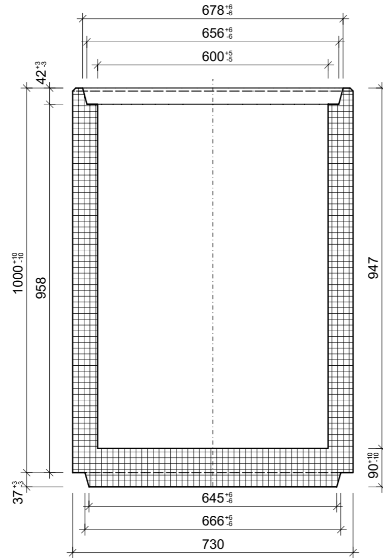
Schnitt 1-1, 1:10
