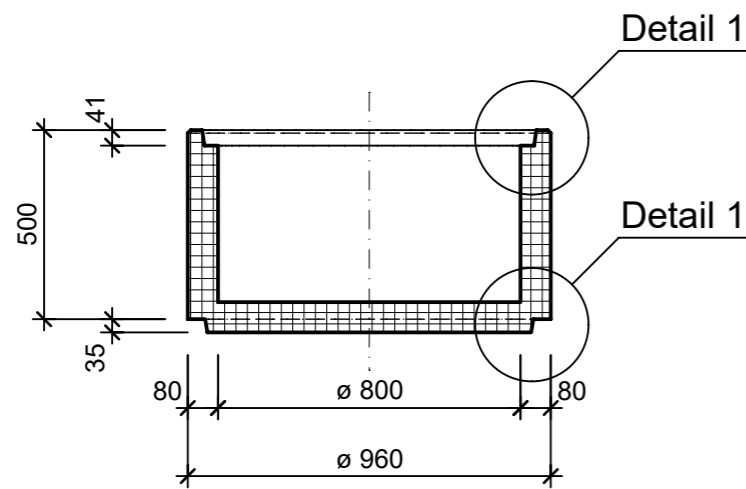
Schnitt A - A, 1:20
