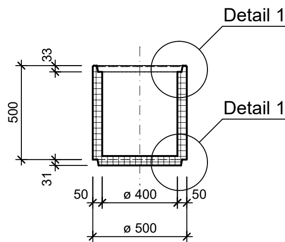
Schnitt A - A, 1:20
