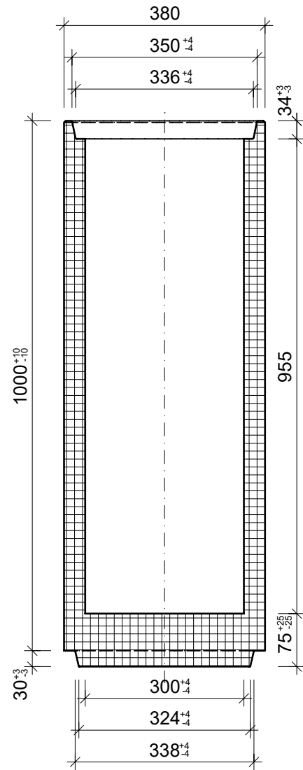
Schnitt 1-1, 1:10
