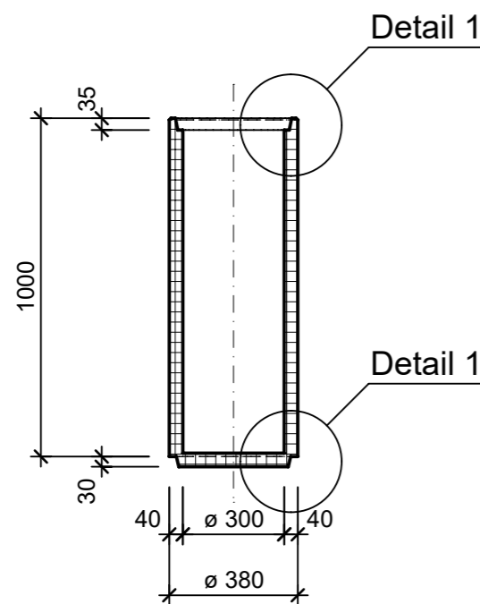
Schnitt A - A, 1:20
