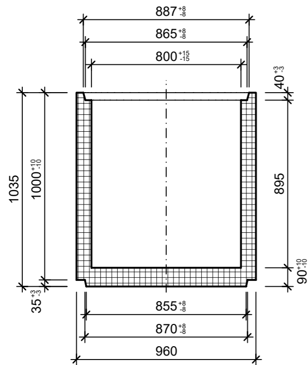
Schnitt 1-1, 1:20
