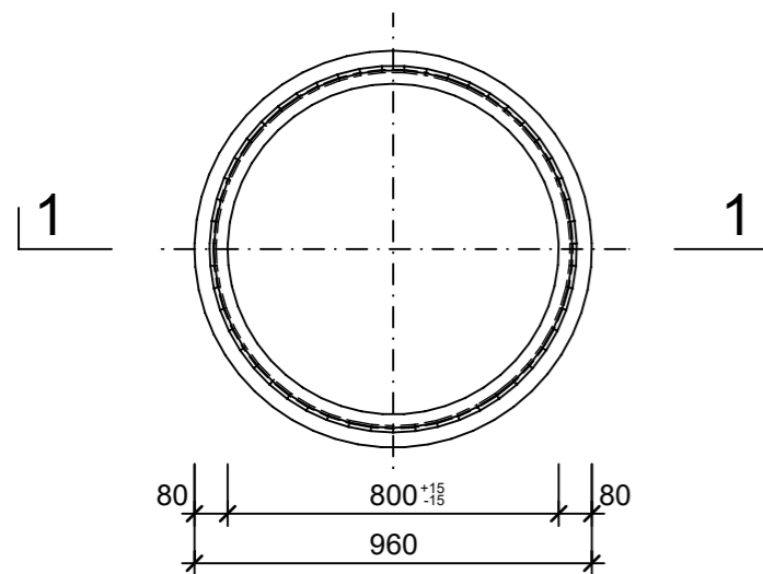
Grundriss, 1:20
