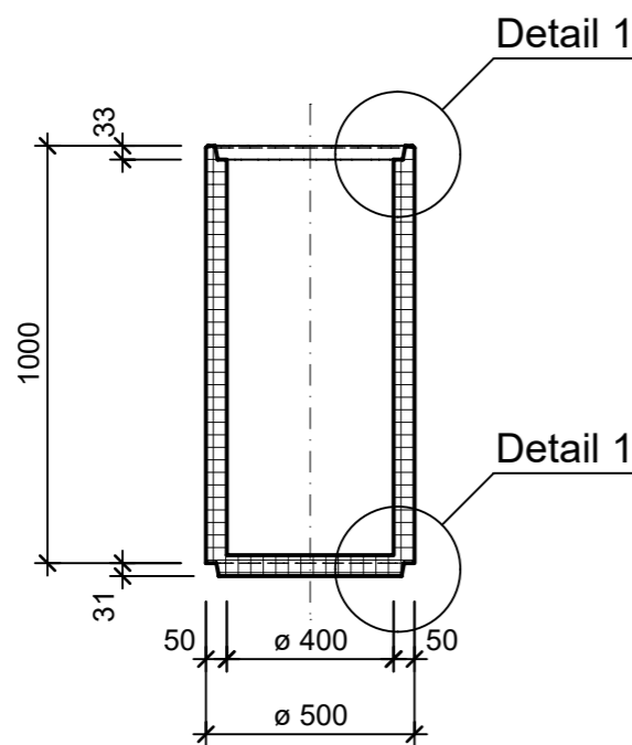
Schnitt A - A, 1:20
