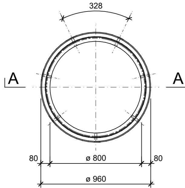
Grundriss, 1:20
