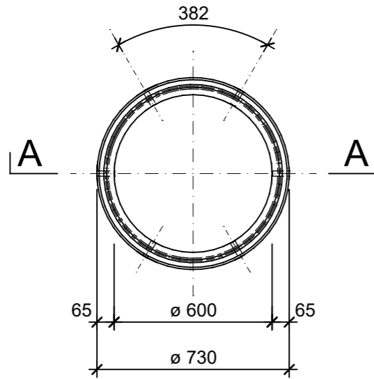
Grundriss, 1:20
