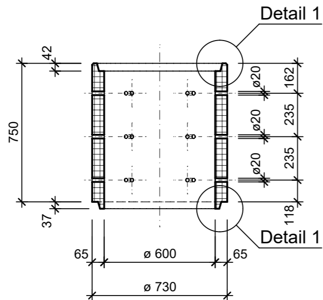
Schnitt A - A, 1:20
