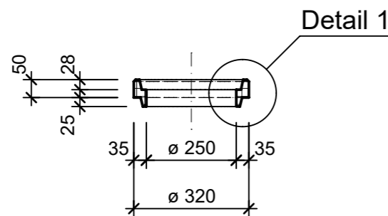
Schnitt A - A, 1:15
