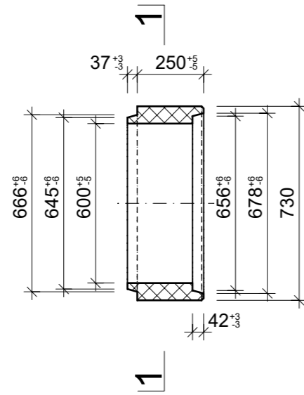
Grundriss, 1:20
