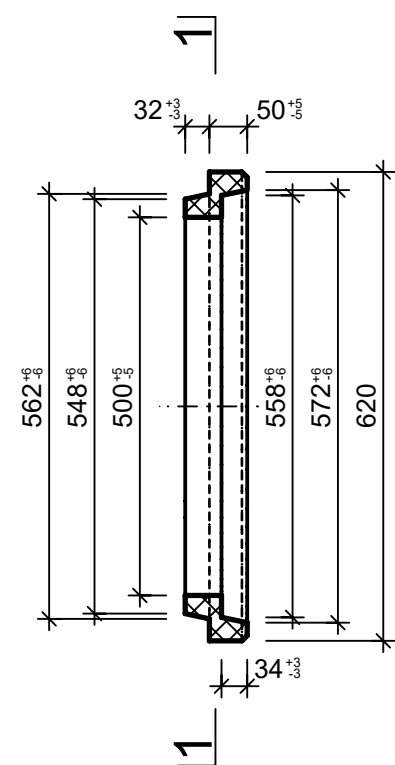
Grundriss, 1:10
