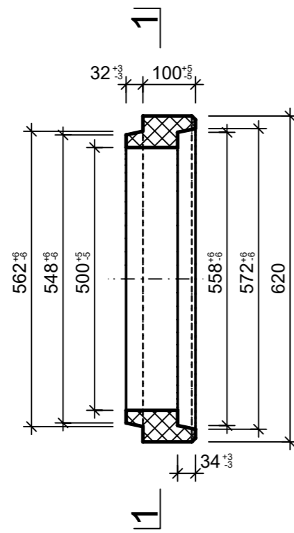
Grundriss, 1:10
