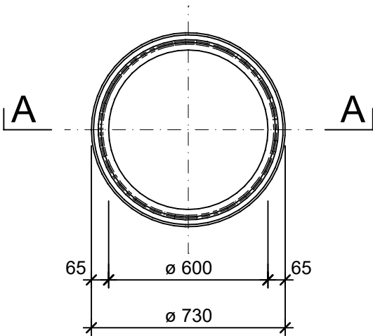
Grundriss, 1:20
