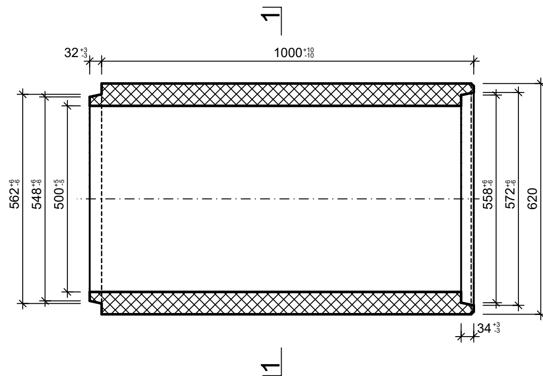
Grundriss, 1:10
