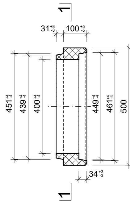
Grundriss, 1:10
