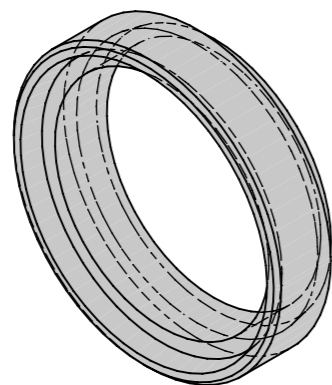
Isometrie, 1:10
