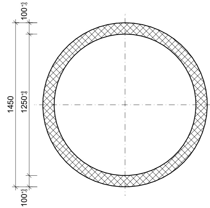
Schnitt 1-1, 1:20
