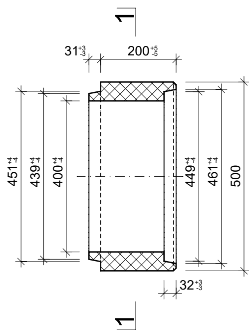
Grundriss, 1:10
