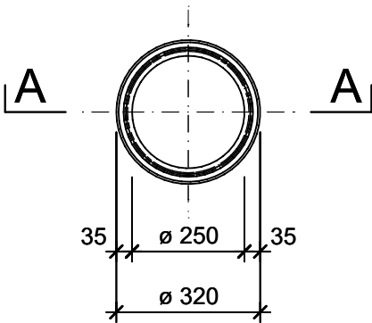
Grundriss, 1:15
