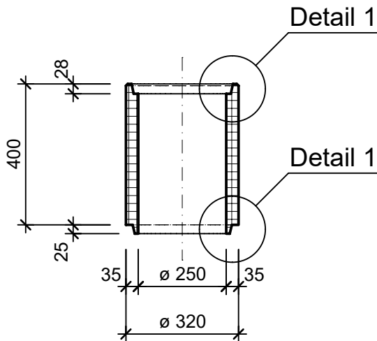
Schnitt A - A, 1:15
