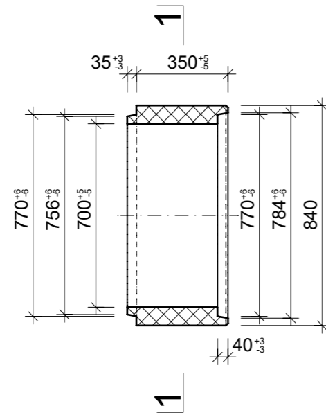
Grundriss, 1:20
