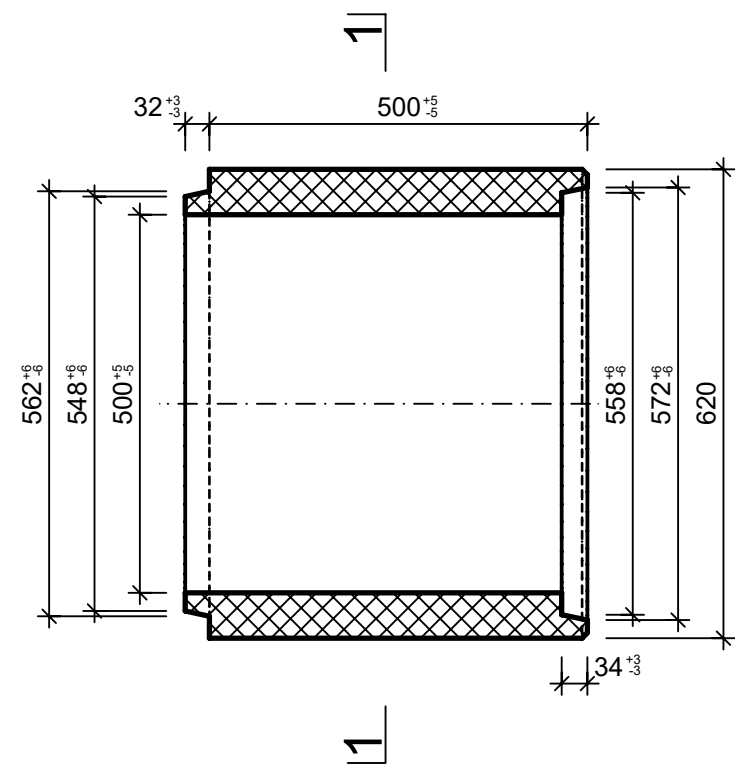
Grundriss, 1:10
