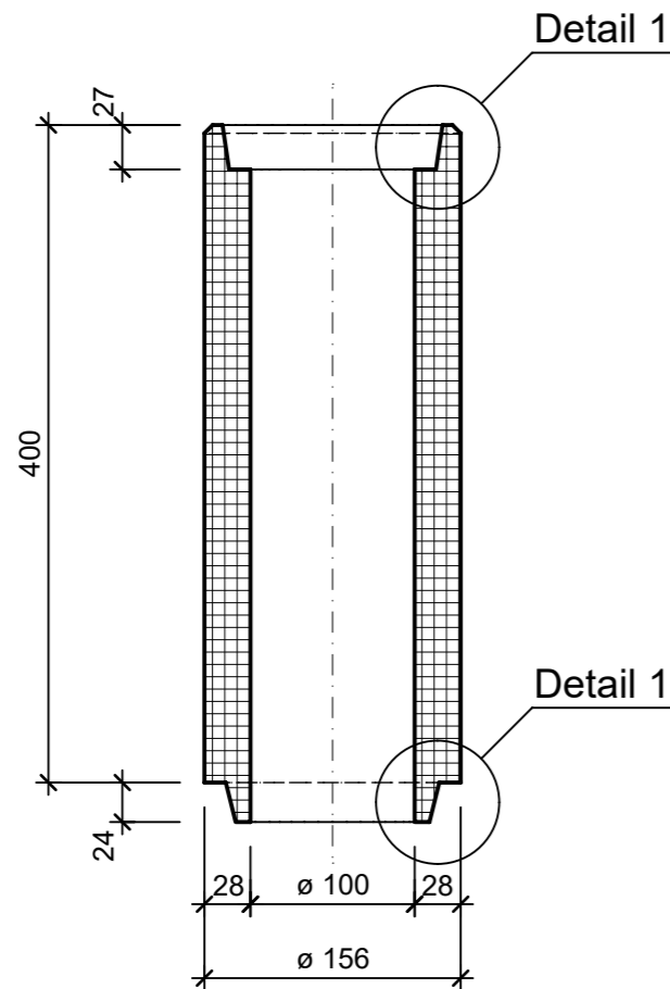
Schnitt A - A, 1:5
