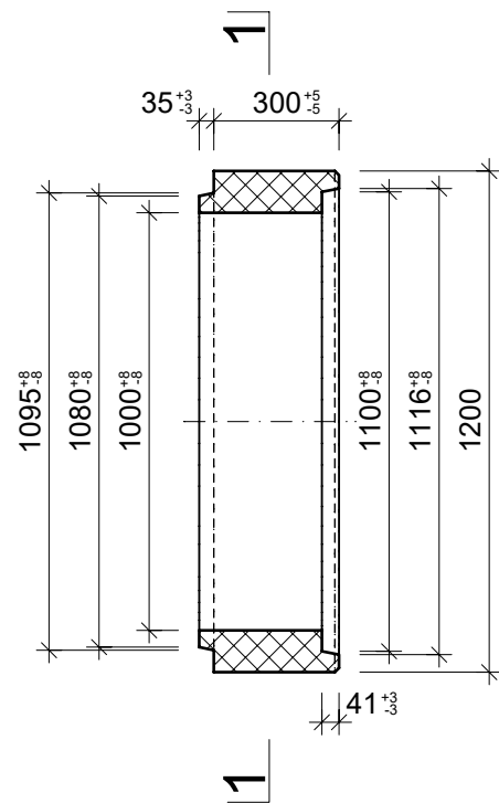
Grundriss, 1:20
