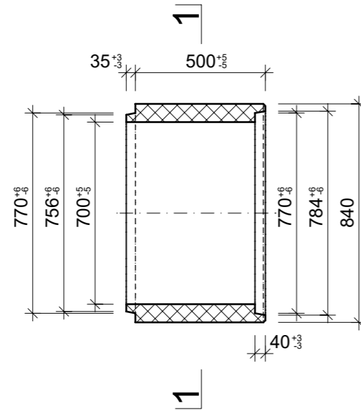
Grundriss, 1:20
