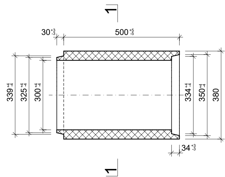
Grundriss, 1:10
