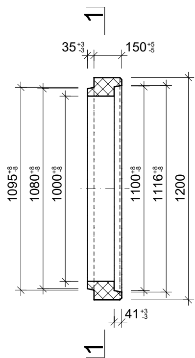
Grundriss, 1:20
