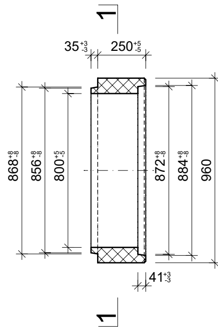
Grundriss, 1:20
