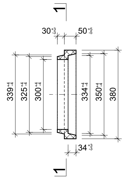
Grundriss, 1:10
