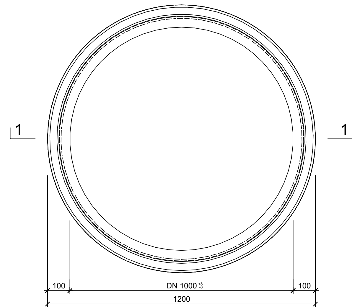
Grundriss, 1:10
