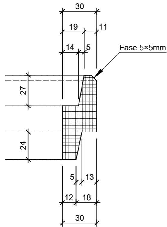
Detail 1, 1:2
