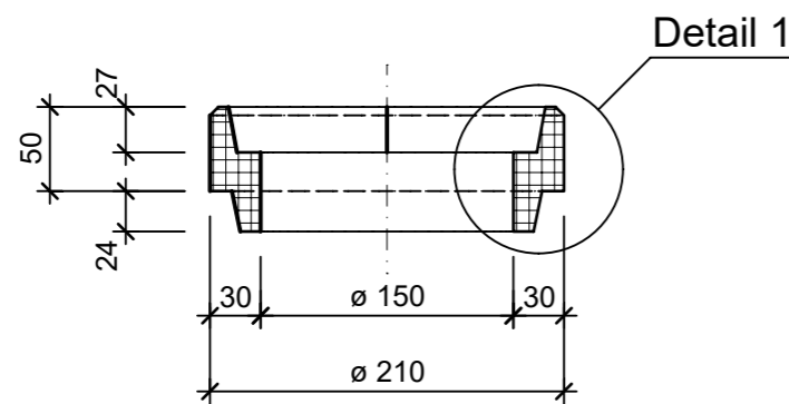
Schnitt A - A, 1:5
