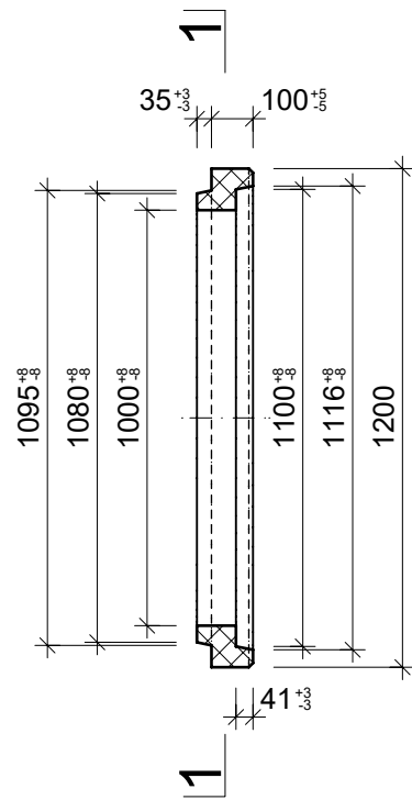
Grundriss, 1:20
