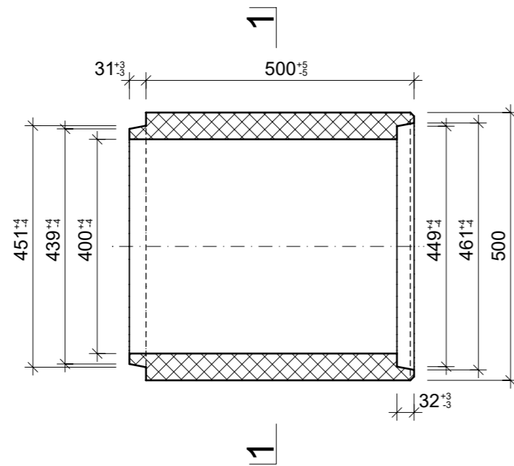
Grundriss, 1:10
