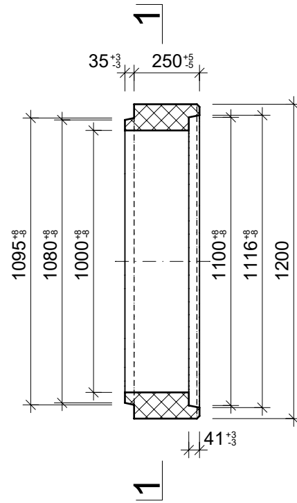
Grundriss, 1:20
