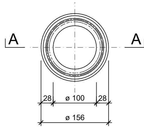
Grundriss, 1:5
