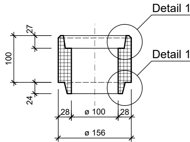
Schnitt A - A, 1:5
