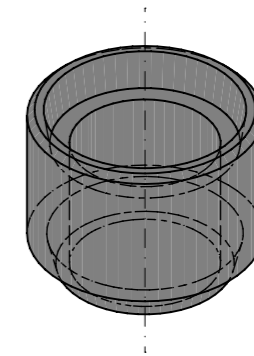
Isometrie, 1:5
