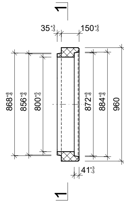
Grundriss, 1:20
