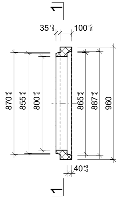
Grundriss, 1:20
