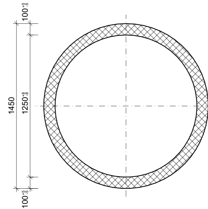
Schnitt 1-1, 1:20
