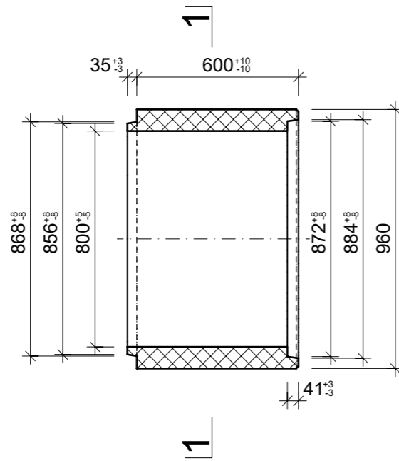
Grundriss, 1:20
