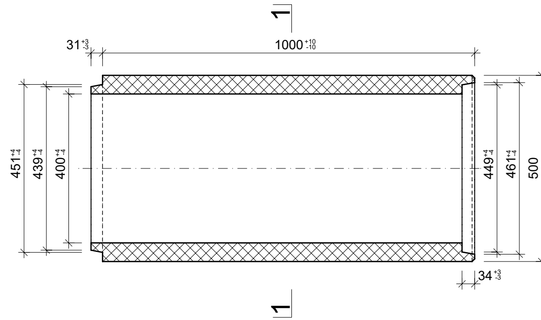
Grundriss, 1:10
