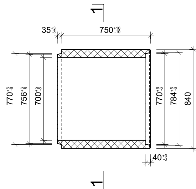
Grundriss, 1:20
