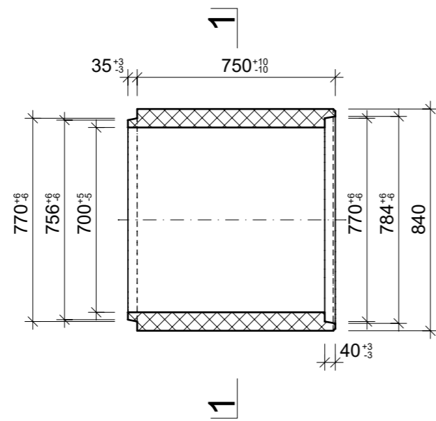
Grundriss, 1:20
