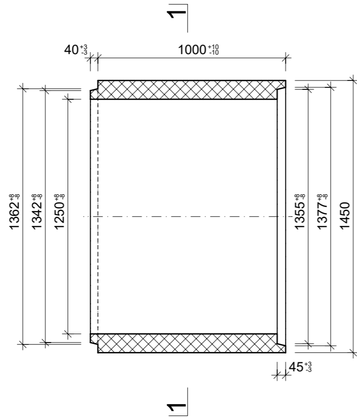
Grundriss, 1:20
